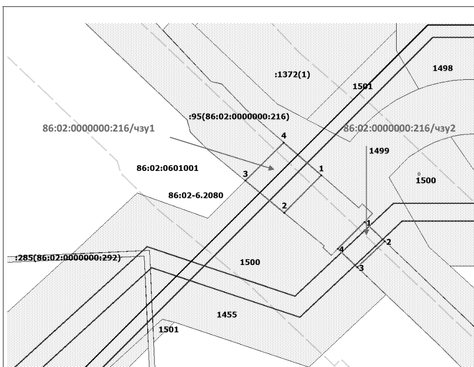
СХЕМА расположения границ публичного сервитута на кадастровом плане территории КК 86:02:0601001
