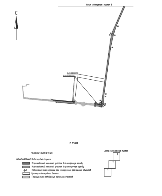
2. Чертеж межевания территории Проект межевания территории для размещения линейного объекта «Причала Приобского региона. Левый берег». Земельный участок: ПАО «НК «Роснефть», Масштаб (1:5000)
