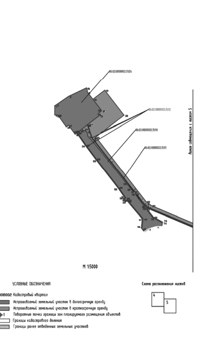
Проект межевания территории для размещения линейного объекта «Причала Приобского региона. Левый берег». Земельный участок: ПАО «НК «Роснефть», Масштаб (1:5000)
